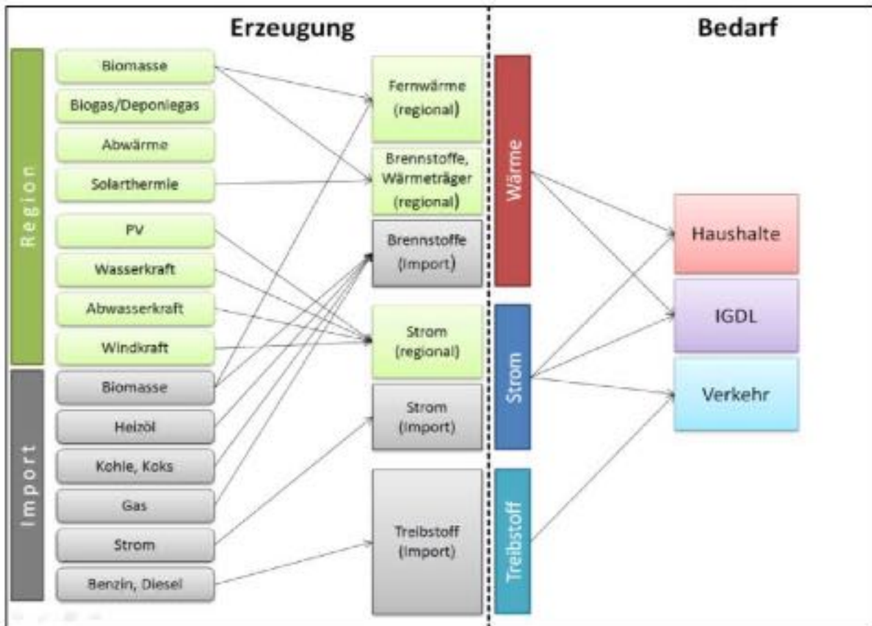
Abbildung 36: Gliederung Energiebilanzmodell
